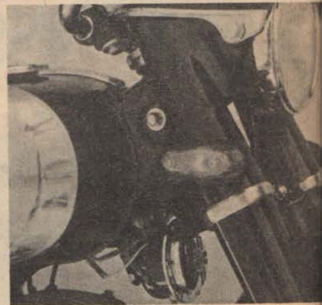
Ci-dessus, avertisseur sous le réservoir, clignotants sur les bras de fourche et phare capoté. Ci-dessous, la suspension avant de la « Benly » rappelle la solution Adler. Notons les butées de caoutchouc.
